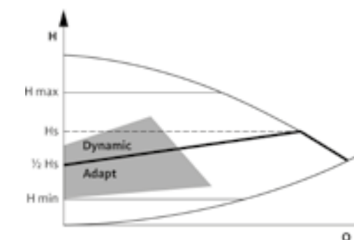
Способ регулирования Др–v с Dynamic Adapt
