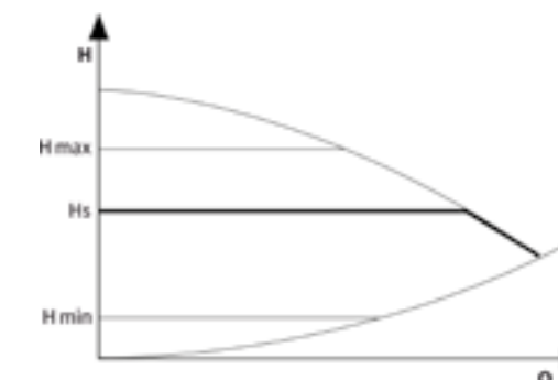
Способ регулирования Др–с
