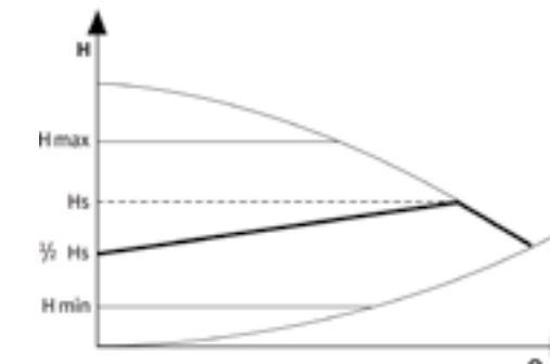
Способ регулирования Др–v
