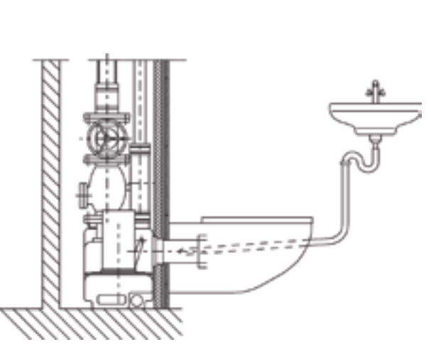
Подключение подвесного унитаза и раковины
